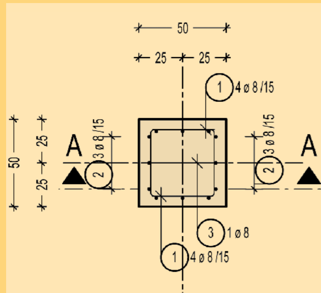
Grundriss
